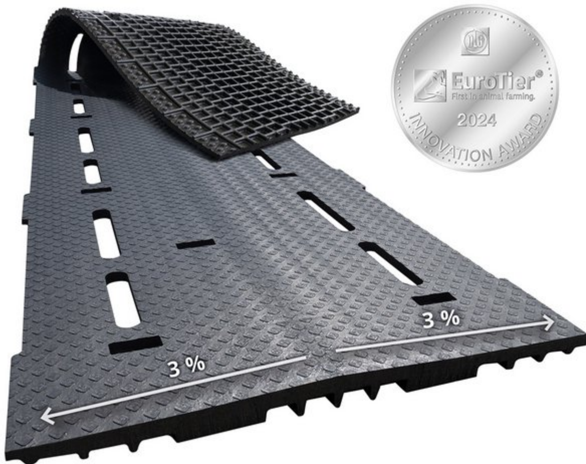
Spaltenmatte espaFLEX mit beidseitigem Gefälle und flexibel gestaltbarem Schlitzbild © KRAIBURG Elastik
