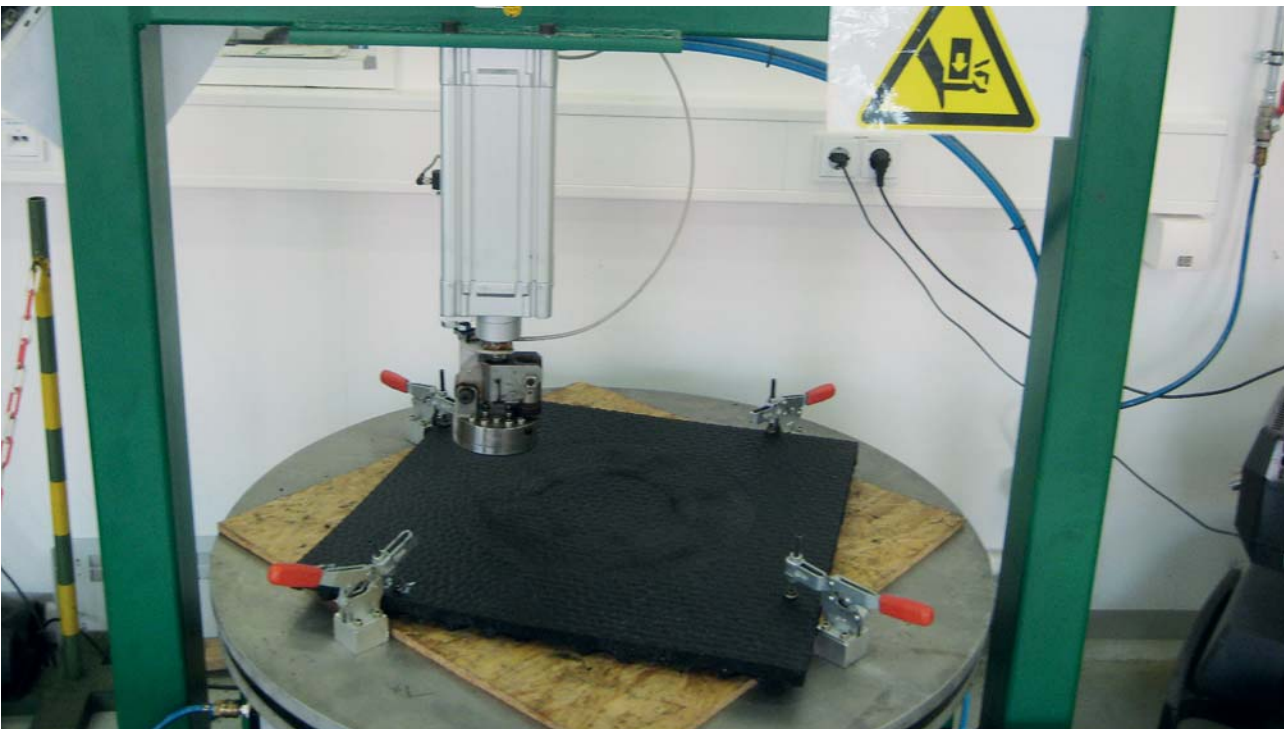
Bild 4: Dauertrittbelastung
