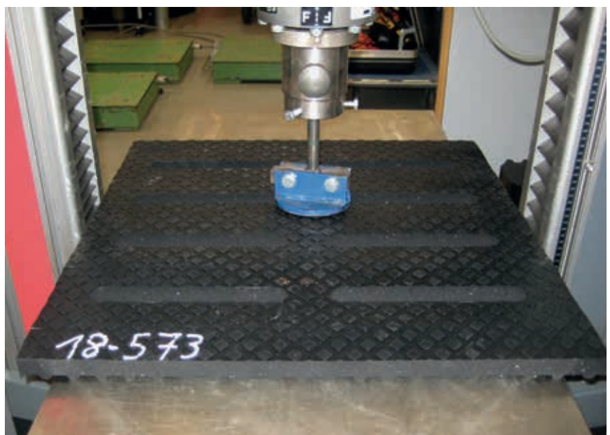
Bild 2: Messung der Verformbarkeit mit Kuhfuß
