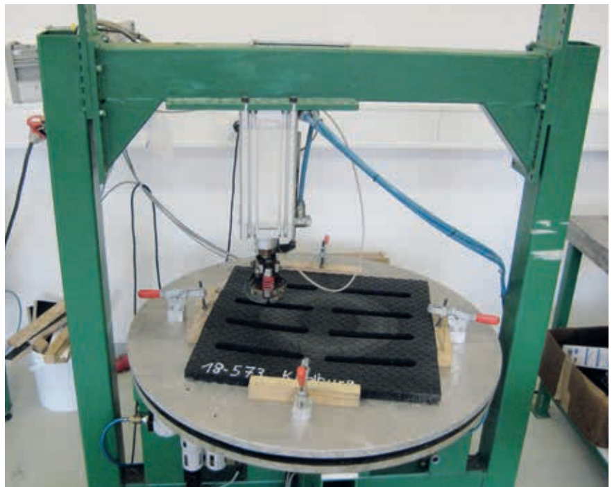
Bild 4: Dauertrittbelastung
