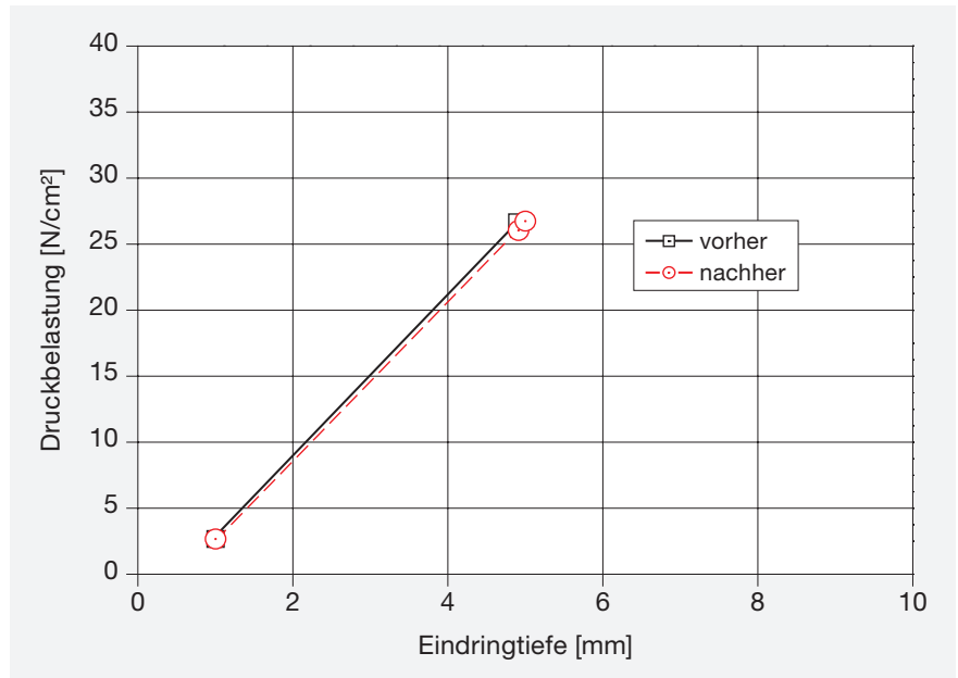
Bild 3: Verformbarkeit in Abhängigkeit vom Auflagedruck vor und nach der Dauertrittbelastung
